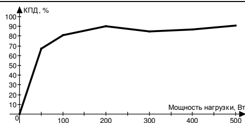
Рисунок 4.1. График зависимости КПД модуля расширения WEM-21xx от мощности нагрузки 1 .
